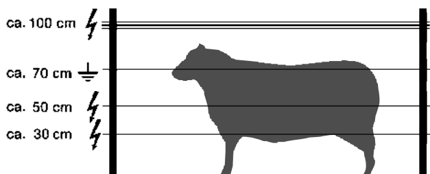
Elektrozaun für Schafe
